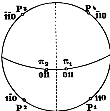
Fig. 3. Zonenverband von i - \alpha -Benzoylmethylhexanonoxim. Monoklin holoedrisch.
